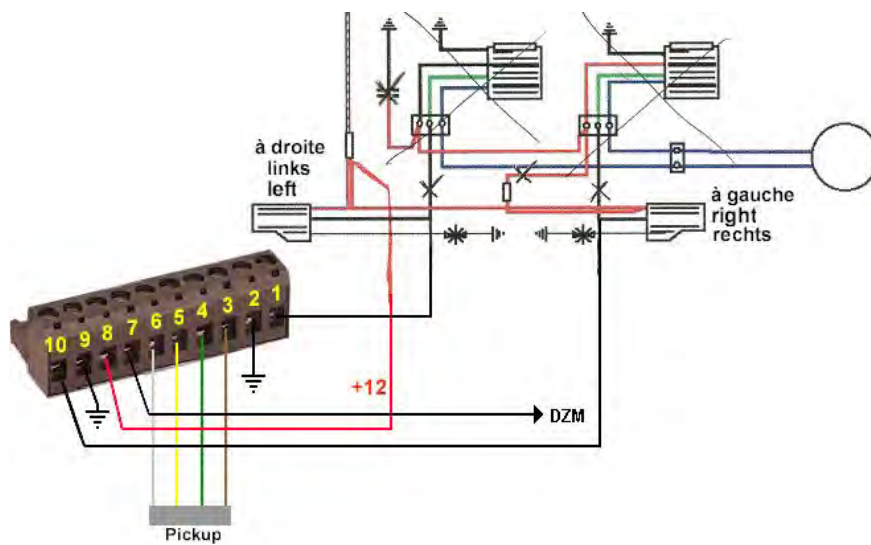
Anschlusschema der Zündung bei Motoplat-Ersatz
