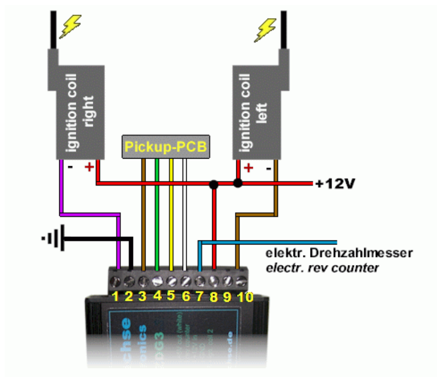
Anschlusschema der Zündung bei Kontakt-Ersatz
