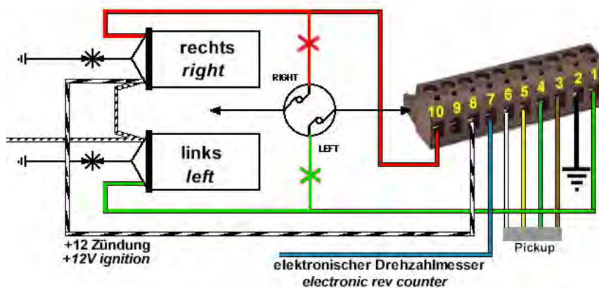
Abbildung 3 Anschlußschema der Zündung bei Kontaktersatz
