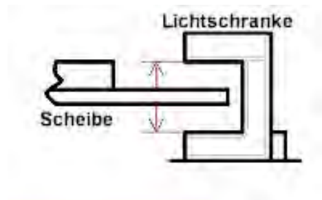
Abbildung 6 Ausrichtung von Sektorscheibe und Lichtschranke.
