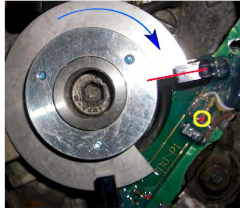
Abbildung 5 Ausrichten der Sektorscheibe so daß die LED gerade an- bzw. ausgeht.
